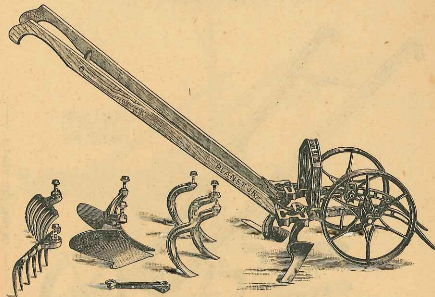
Planet jun. Doppelrad-Hacke.
